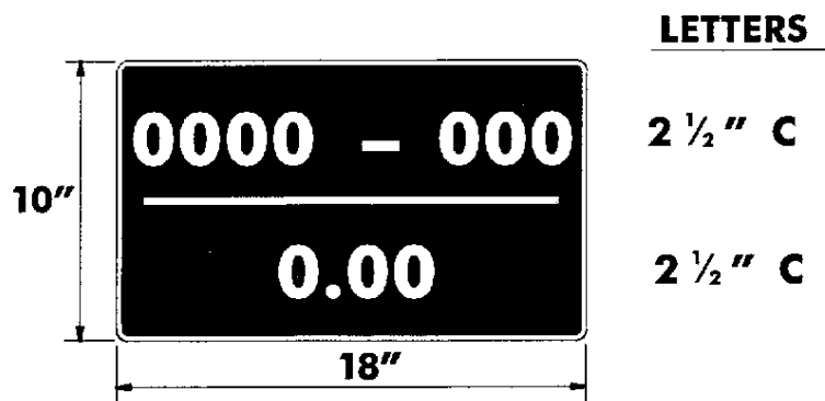
D(NJ)13-1
